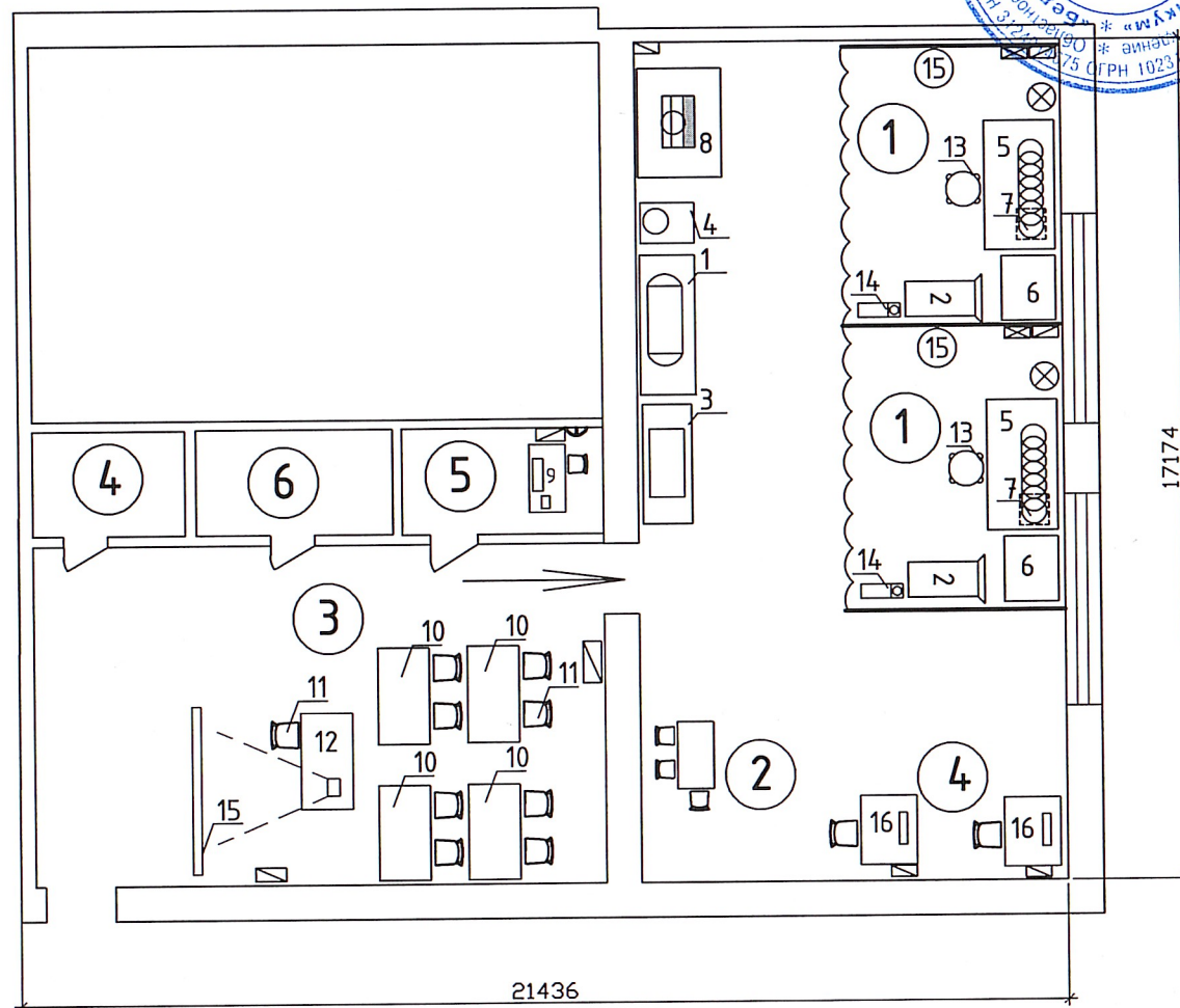
План застройки Мастерская "Обработка листового металла "
